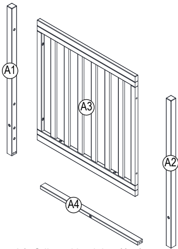
A: Crib End (1 pc)
